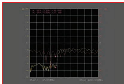
2 Satellite: Αντίστοιχα η προσαρμογή της περιοχής της δορυφορικής λήψης. Εδώ συνοπολογίστε +6 dB στην κίτρινη ένδειξη για την απώλεια ενός DC inserter που κάναμε χρήση για να στείλουμε την εντολή στο multiswitch.
